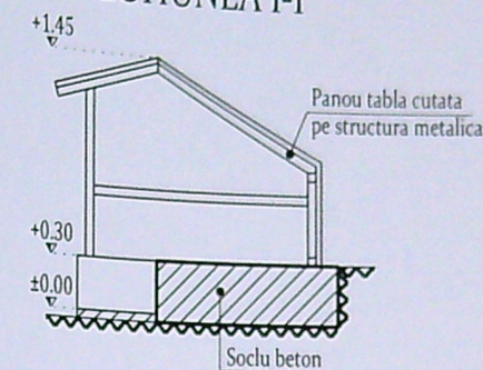
SECTIUNEA 1-1
